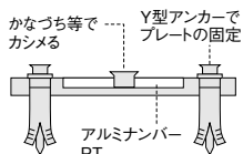
左矢タイプ A325LT2
