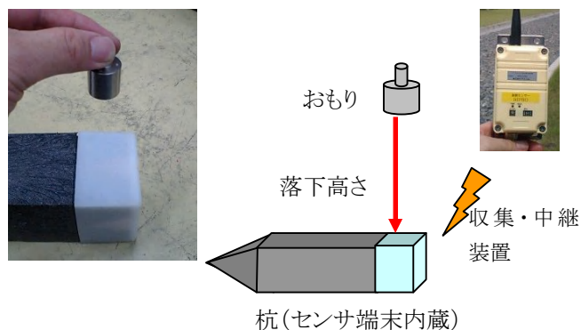
図-7 落下によるセンサ検知の確認
