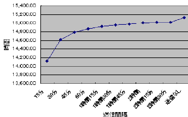
図-4 通信頻度と電源の寿命の関係（概算）
