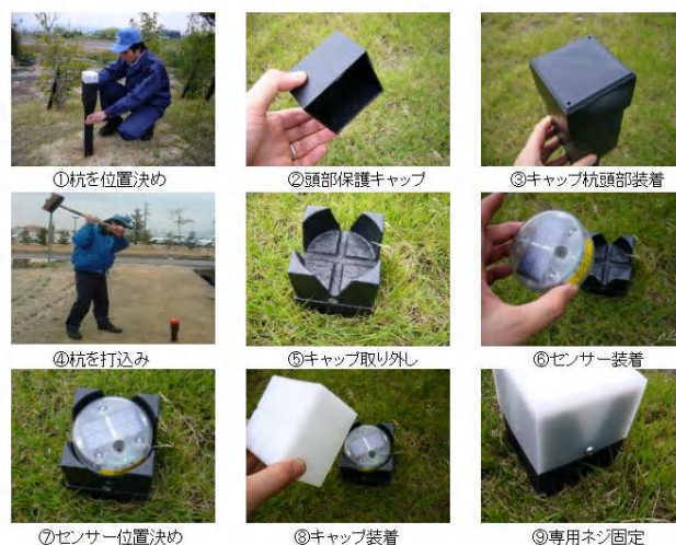
図-5 杭設置（打ちこみ）の手順
